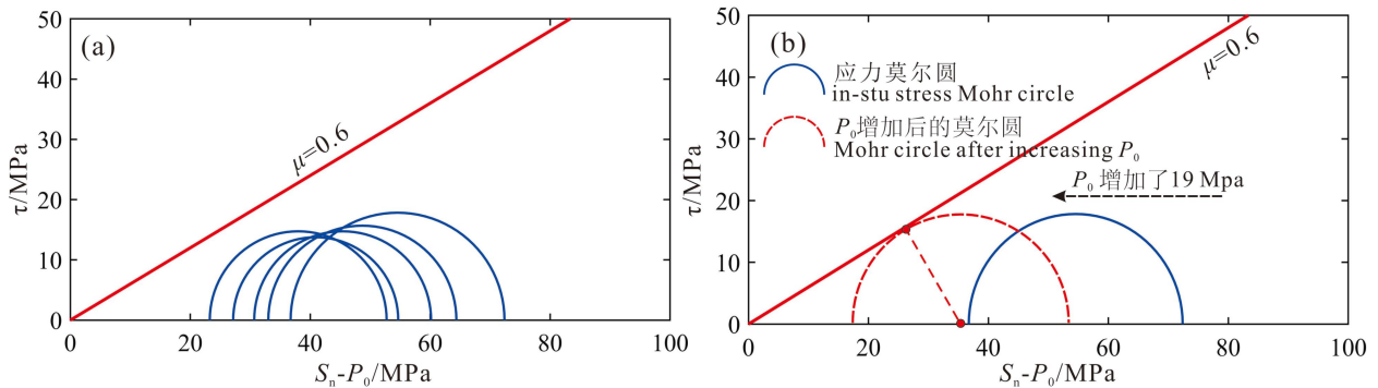
a—基于地应力的莫尔圆断层活动性分析；b—GR2 井在 4500 m 处断层随孔隙压力的增加可能导致不稳定
