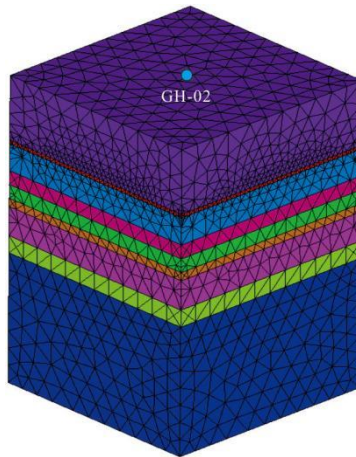
图 5 干热岩研究区三维有限元网格模型
