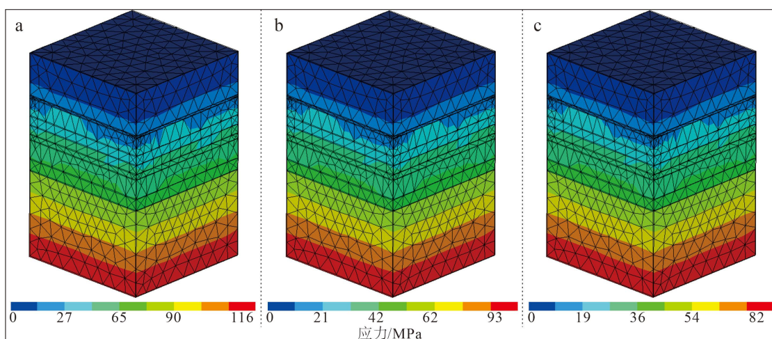
图 6 干热岩研究区三维主应力云图
