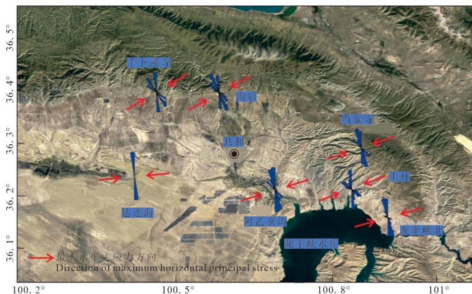
图2 基于裂隙统计的共和干热岩区地应力方向投影图(据雷治红, 2020修改)
