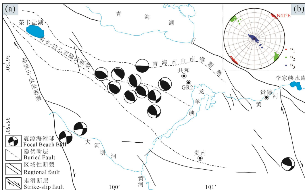
图4 共和盆地震源分布图(a)（据雷治红，2020修改）和震源机制综合解(b)
