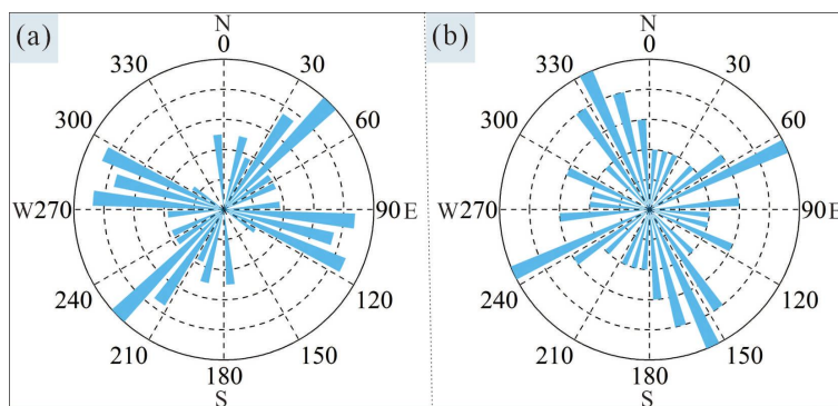
图3 共和盆地干热岩区最大水平主应力方位(据王洪等, 2021修改)
