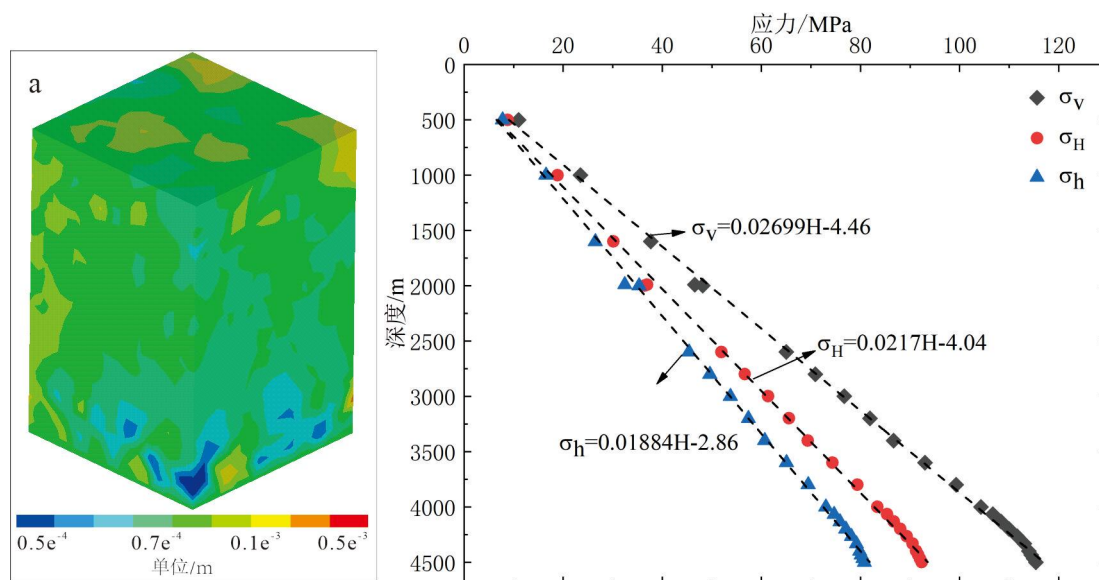
图 7 干热岩 GR2 井位移、地应力模拟结果图
