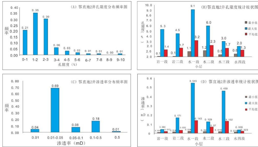
图 4 鄂宜地 2 井岩家河-水井沱组 (A) 孔隙度分布频率图; (B) 各小层孔隙度统计图; (C) 渗透率分布频率图; (D) 各小层渗透率统计图.
