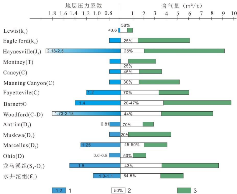
图 11 典型区块页岩含气性、赋存状态及与地层压力间关系 (据 Hill, 2000; 有修改)
