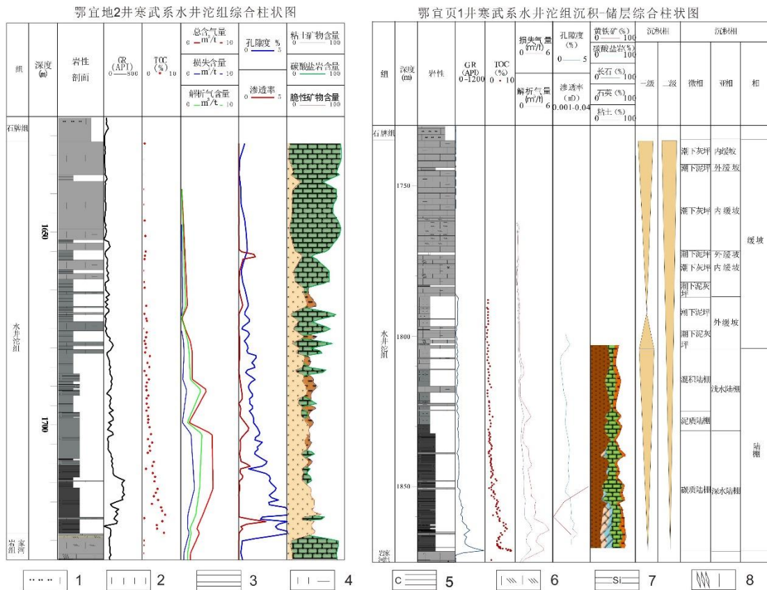
图2 宜昌地区鄂宜页1井和鄂宜地2井沉积-储层综合柱状图
