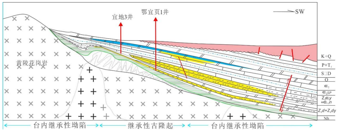
图 12 宜页 1 井寒武系页岩气“基底控藏型”保存模式（据陈孝红等，2018；有修改）
