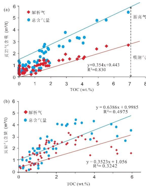
图 8 现场解析含气量与 TOC 关系图
