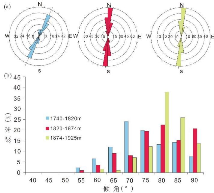
图 10 鄂宜页 1 井水井沱组裂缝分布特征（据罗胜元等，2019；有修改）
