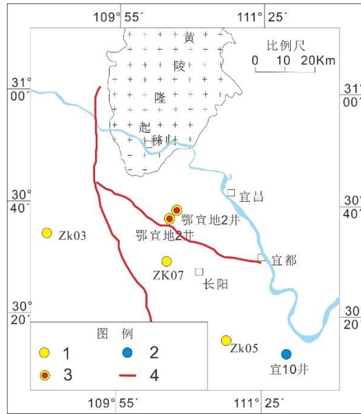
图 1 钻井及钻孔位置分布图 (据罗胜元等, 2022; 有修改)
