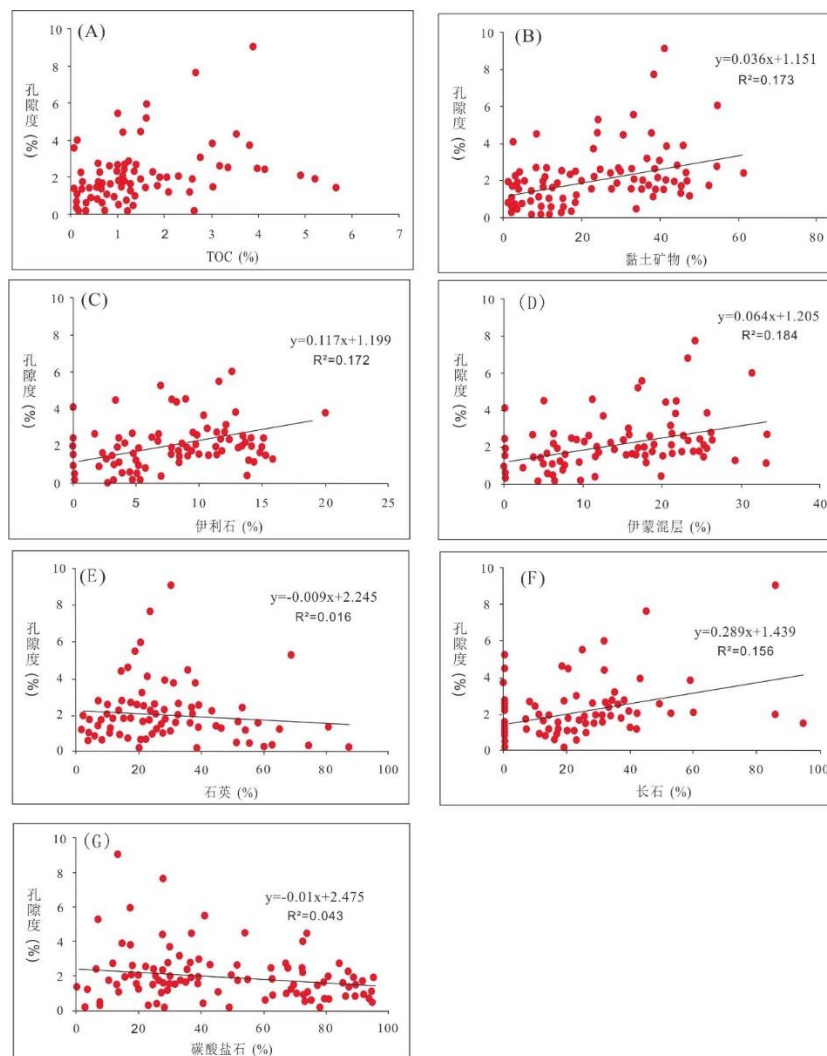
图 7 鄂宜地 2 井水井沱组页岩孔隙度与不同物质含量的关系
